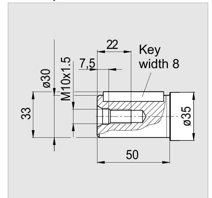
Parallel Keyed Shaft: DIN 6885 8x7x40
